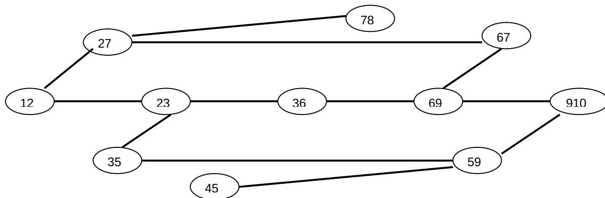
Fig. 3. Transformarea Kaufmann pentru graful considerat al stației din fig. 2
