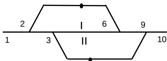
Fig. 10. O stație de cale ferată cu drumuri de alunecare notate conform sensului de parcurgere : I – 6 respectiv II – 3
