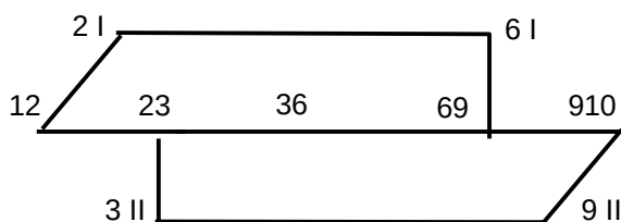
Fig. 11. Transformarea Kaufmann pentru graful stației din fig. 10
