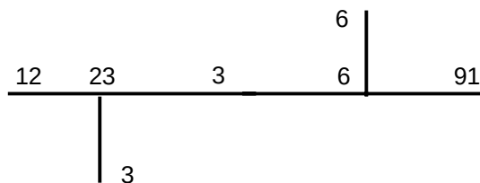
Fig. 13. Transformarea Kaufmann pentru graful stației din fig. 12
