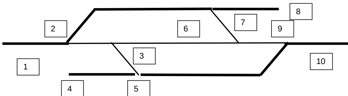
Fig. 6. Parcursurile compatibile determinate matematic (în care evidențierea liniilor mai groase – pentru materializarea parcursurii – a apărut pe măsură ce demonstrația avansa).
