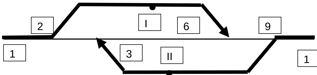
Fig. 14. Parcursurile compatibile determinate matematic (în care necesitatea considerării liniilor mai groase a apărut pe măsură ce demonstrația avansa)
