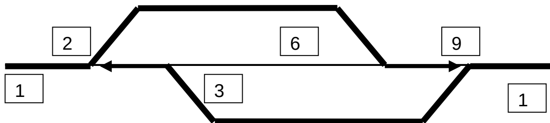
Fig. 9. Cele două parcursurile care nu îndeplinesc condițiile de siguranță a circulației
