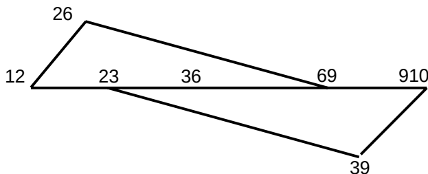
Fig. 8. Transformarea Kaufmann pentru graful considerat al stației din fig. 7
